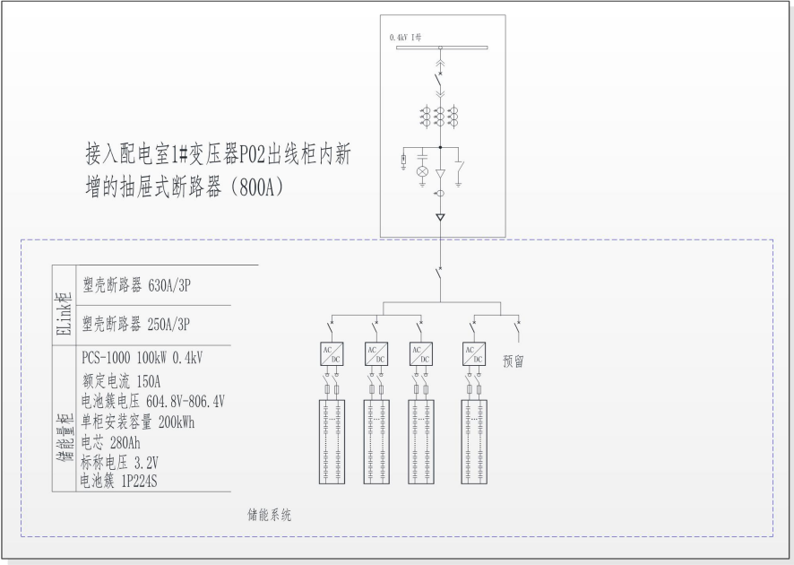
6. 储能接入拓扑图（示范图例）
