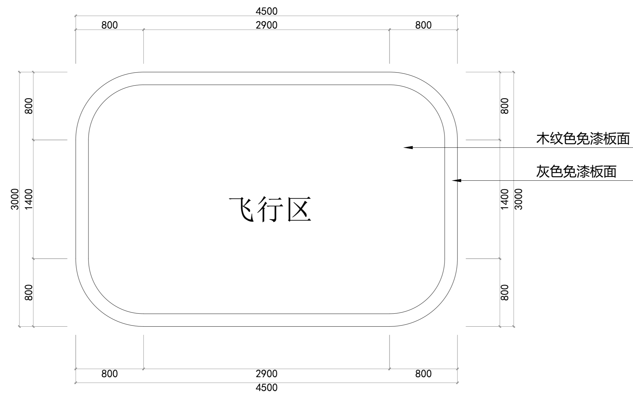
飞行区平面尺寸图
