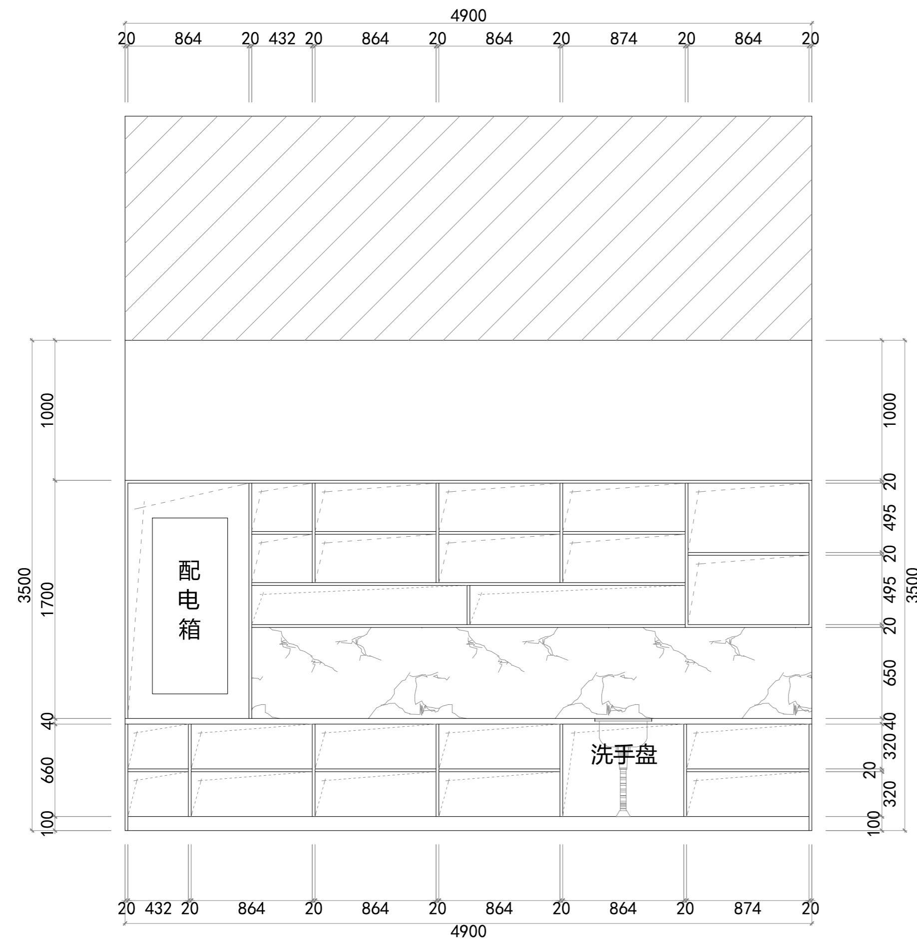
柜内立面图
