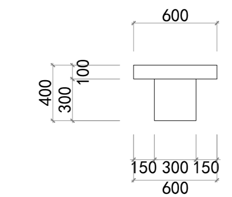
长凳剖面尺寸图
