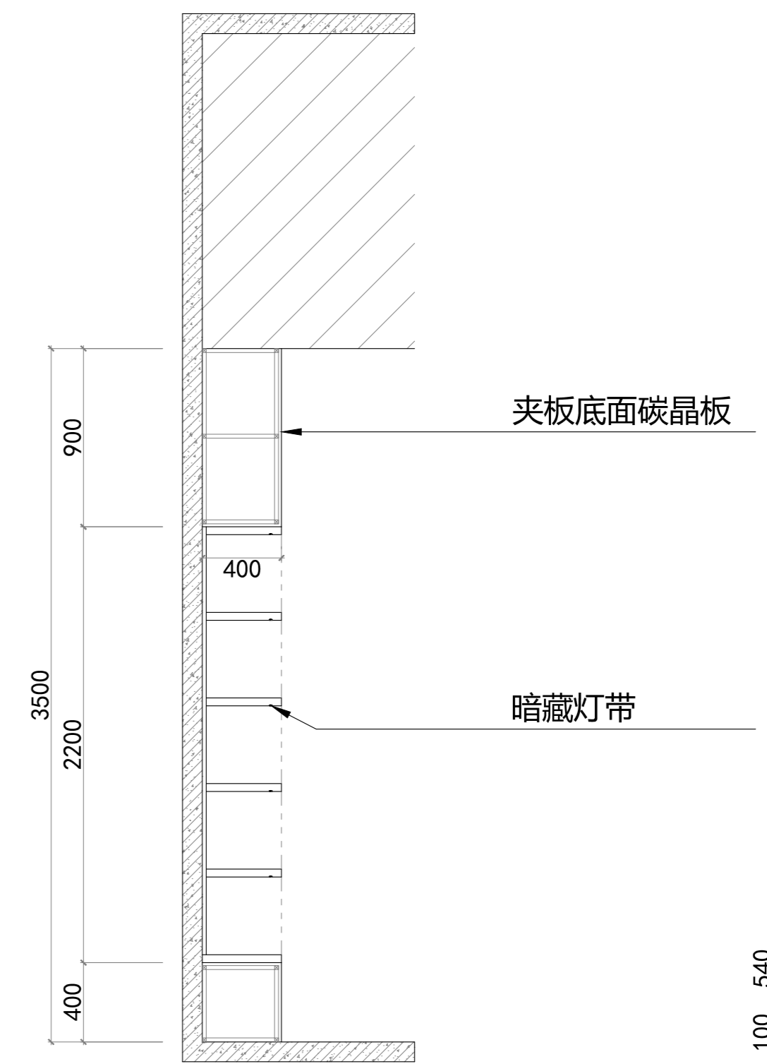
剖面尺寸图
