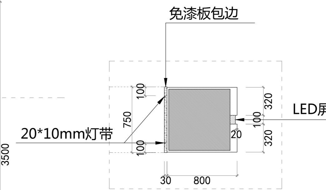
剖面尺寸图
