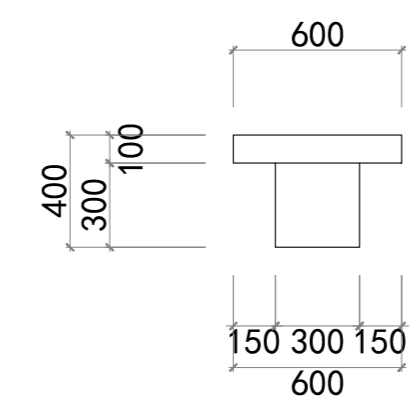
长凳剖面尺寸图
