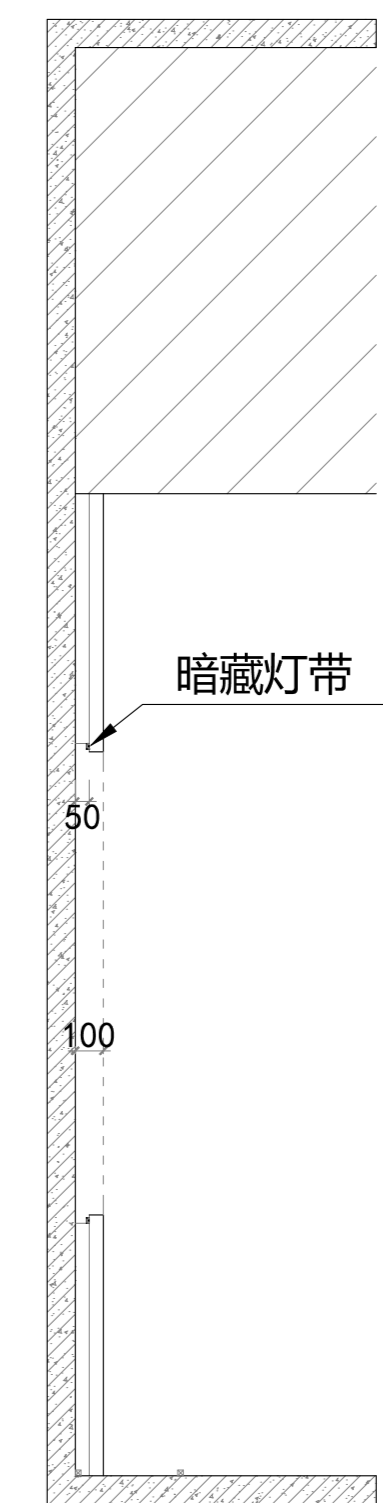
剖面尺寸图
