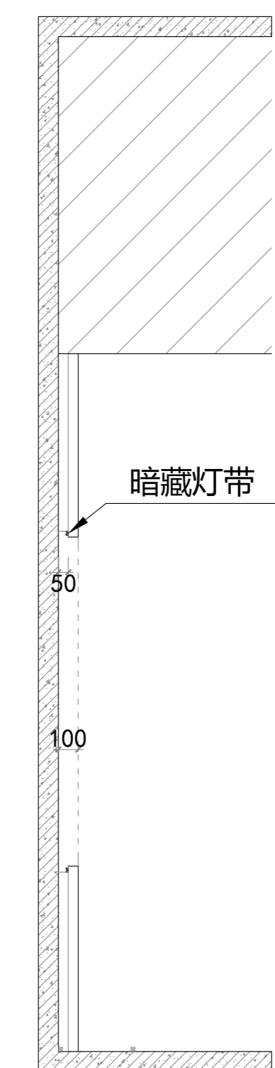
剖面尺寸图
