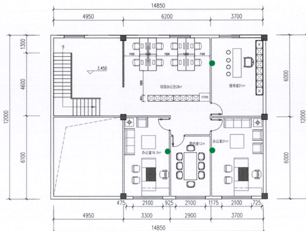
项目指挥部 (临时展厅) 二层平面布置图
