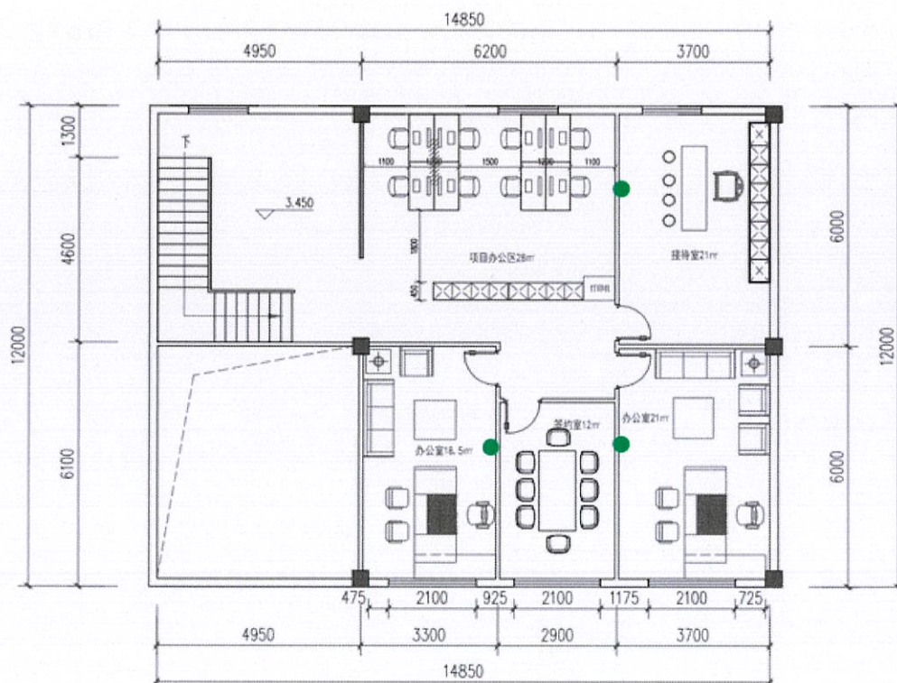
项目指挥部（临时展厅）二层平面布置图
