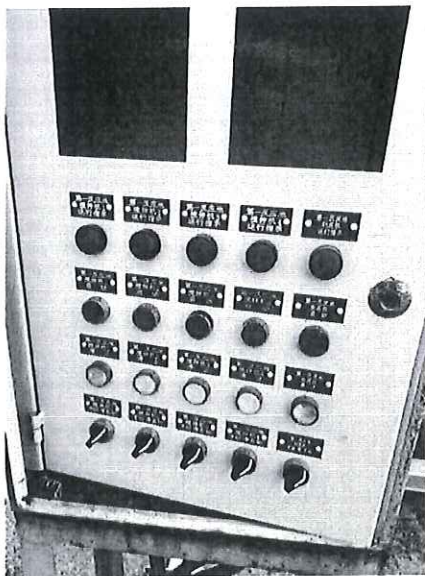
现场按钮箱：
