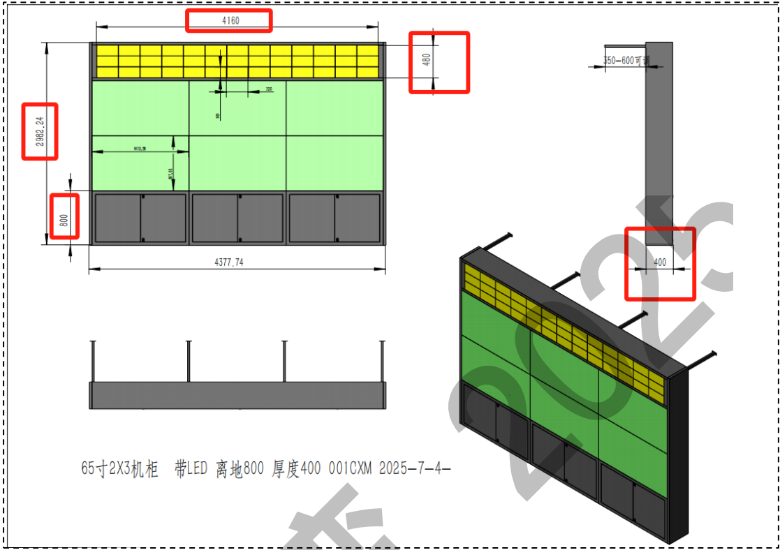
拼接屏配套落地柜示意图
