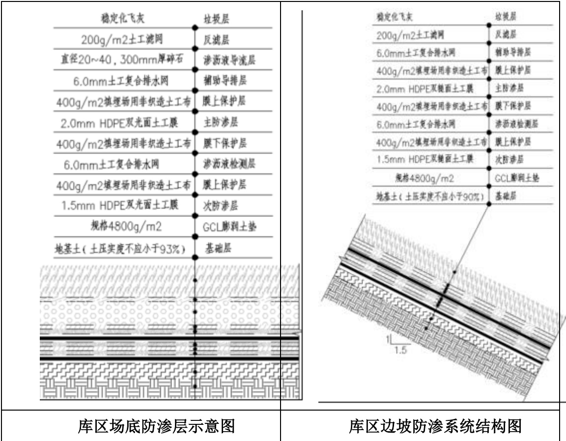
图 3.7-5 填埋场重点污染区防控措施
