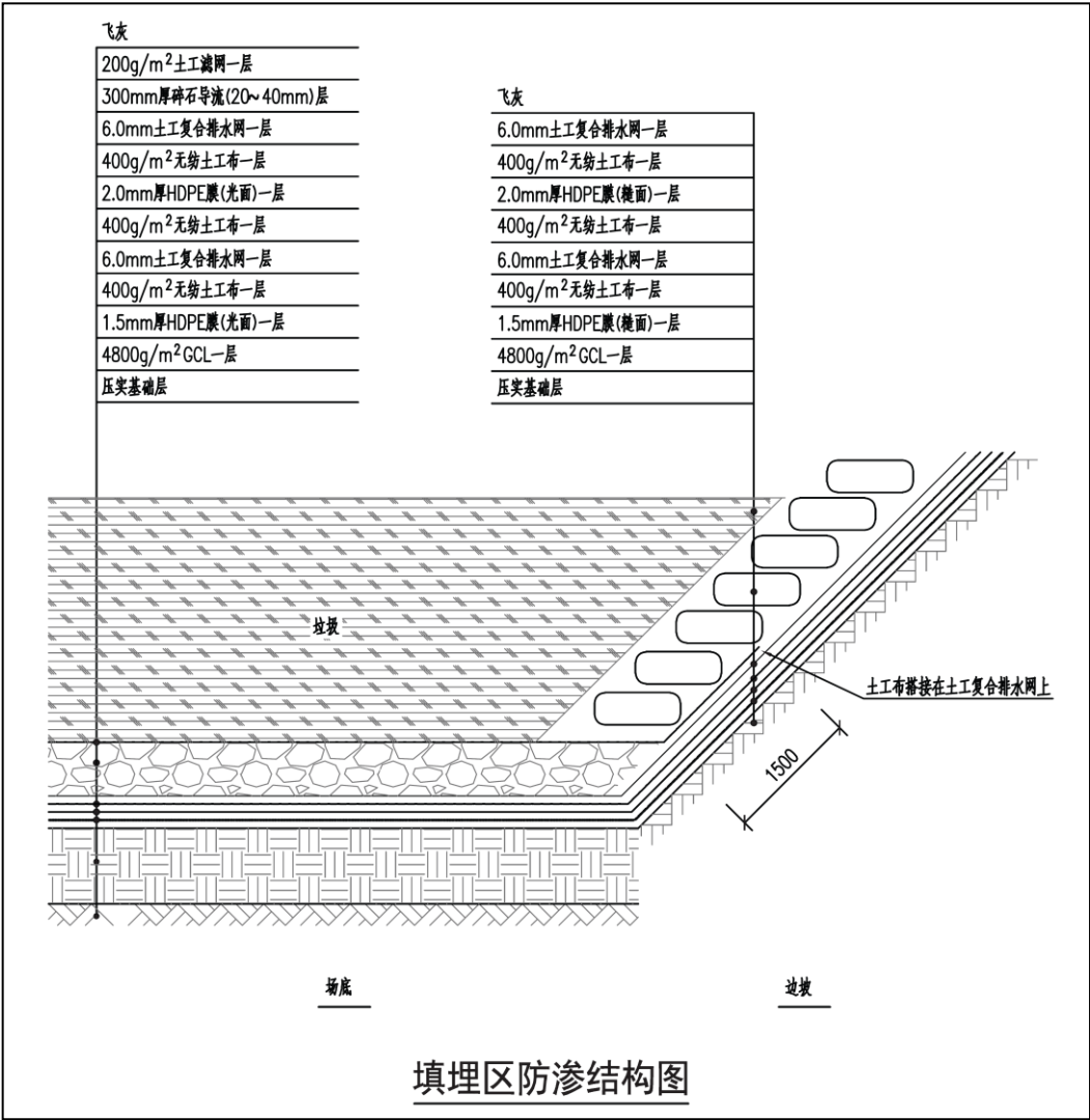
图 4.1-7 填埋区场底及边坡防渗结构图
