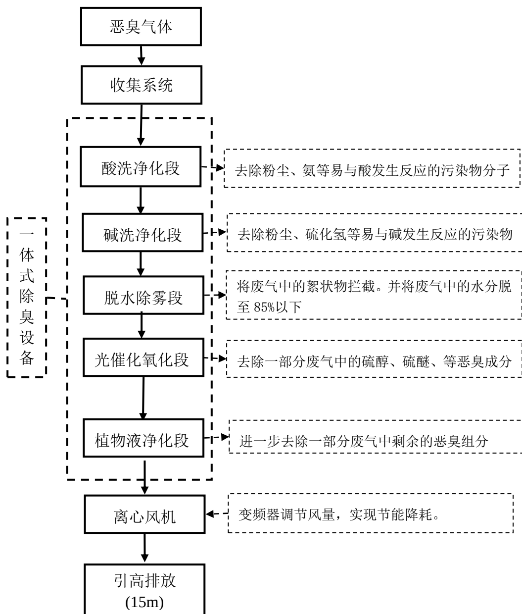
图 7.1-1 除臭系统工艺流程图
