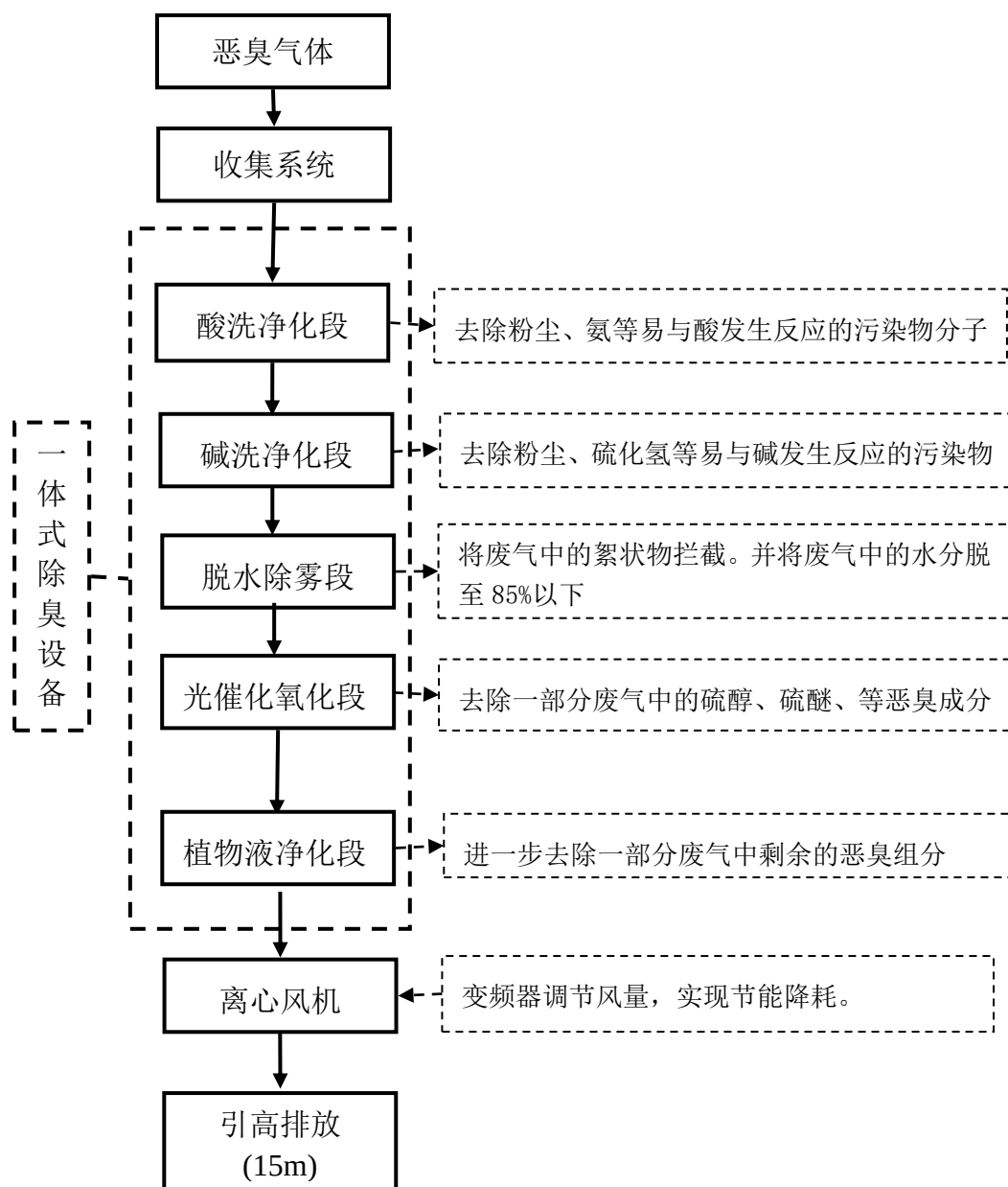
图 3.12-3 除臭系统工艺流程图
