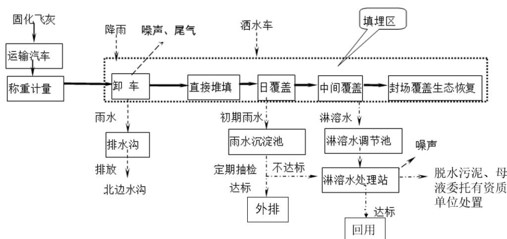
图 4.2-6 飞灰固化体填埋工艺流程及主要产污节点示意图
