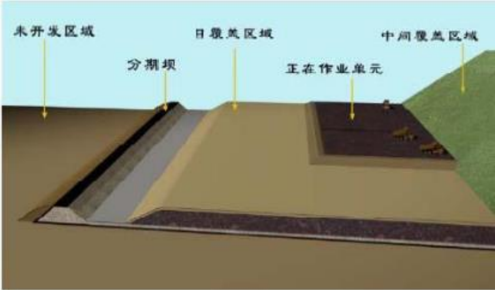
图 3.7-7 雨污分流原理示意图
