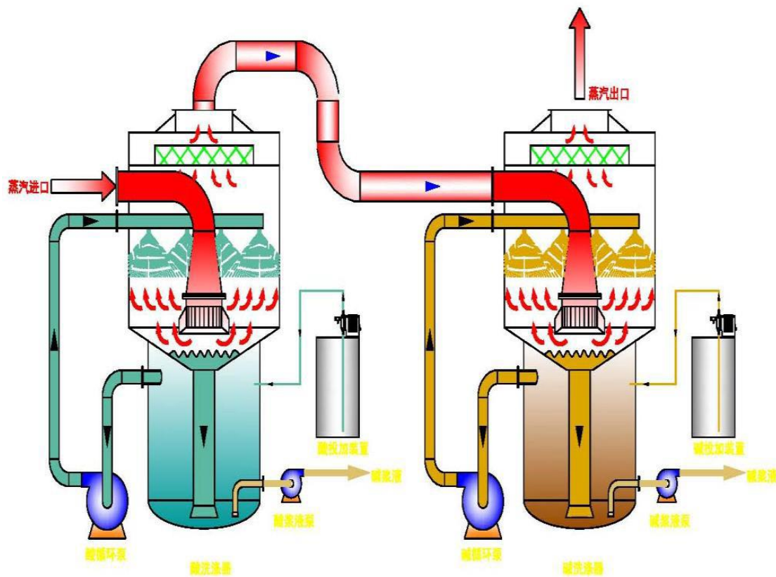
图 3.12-2 酸碱洗气系统示意图
