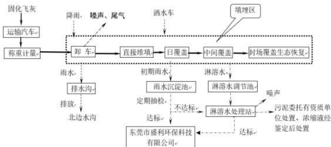
图 3.5-2 飞灰固化体填埋工艺流程及主要产污节点示意图
