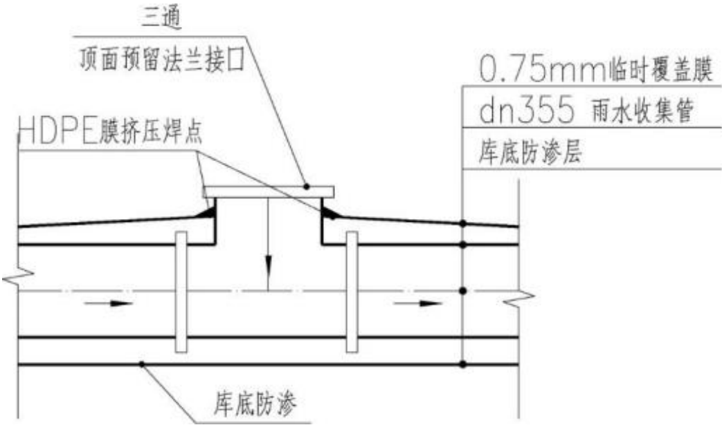
图 3.7-8 膜面雨水收集口
