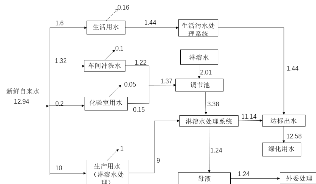
图 4.2-8 拟建项目水平衡图 (m 3 /d)
