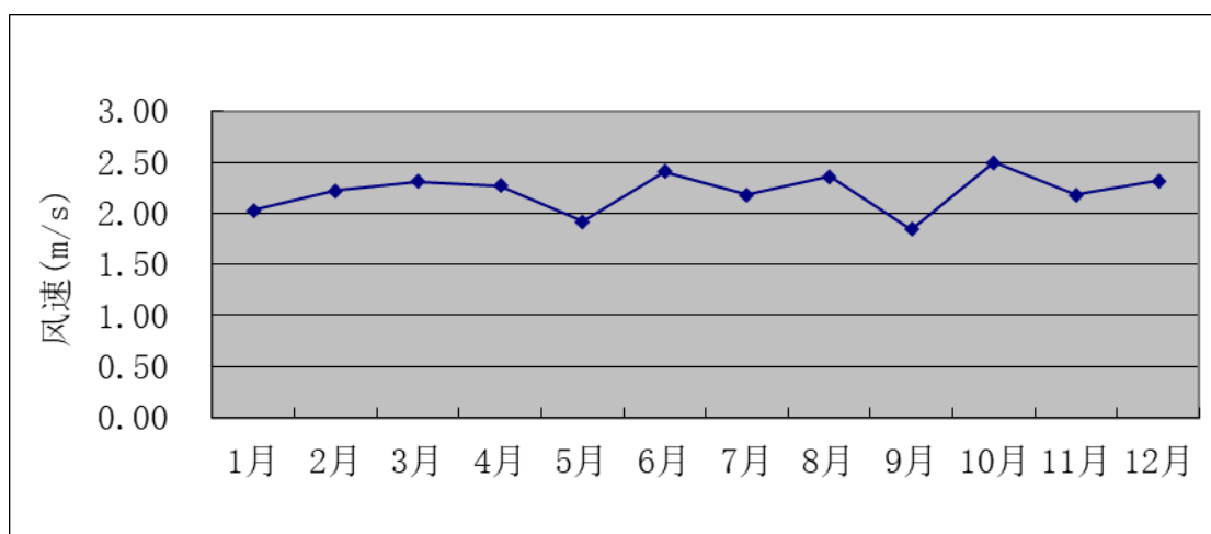
图 6.1-3 年平均风速的月变化图
