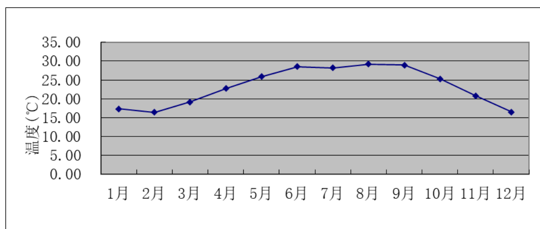
图 6.1-2 年平均温的月变化图
