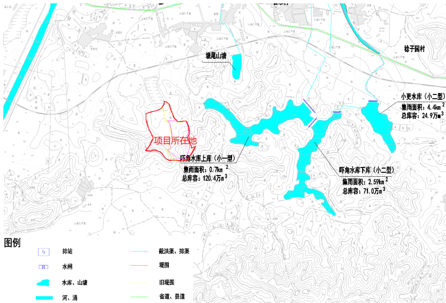
图 2.5-4 项目所在区域水力联系图
