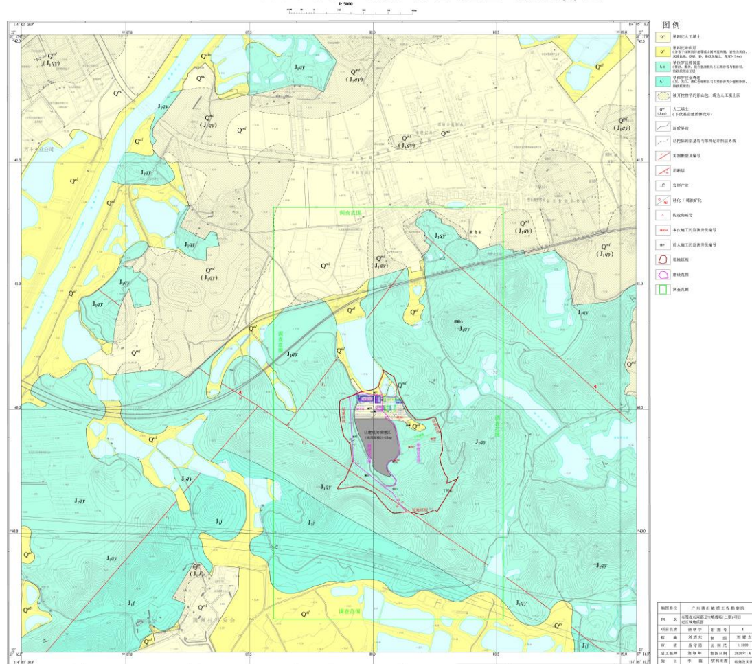
图 6.3-2 项目近区域地质图
