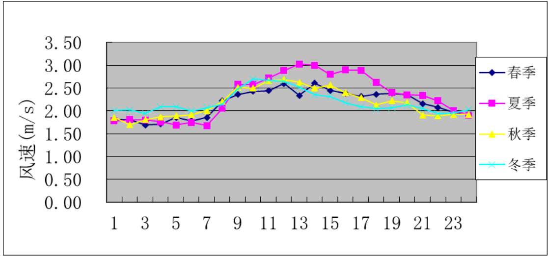
图 6.1-4 季小时平均风速日变化图
