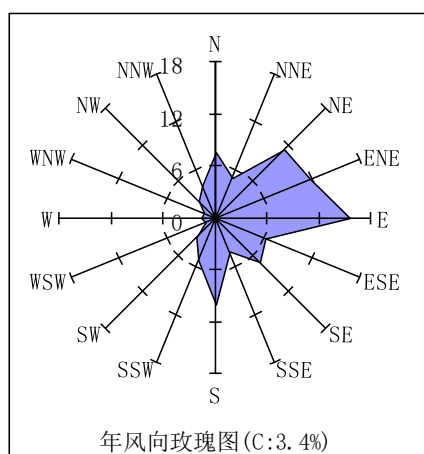
图 6.1-1 东莞气象站风向玫瑰图 (统计年限: 1998-2017 年)
