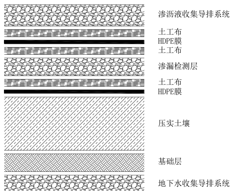
图 4.1-8 双层防渗结构的层次
