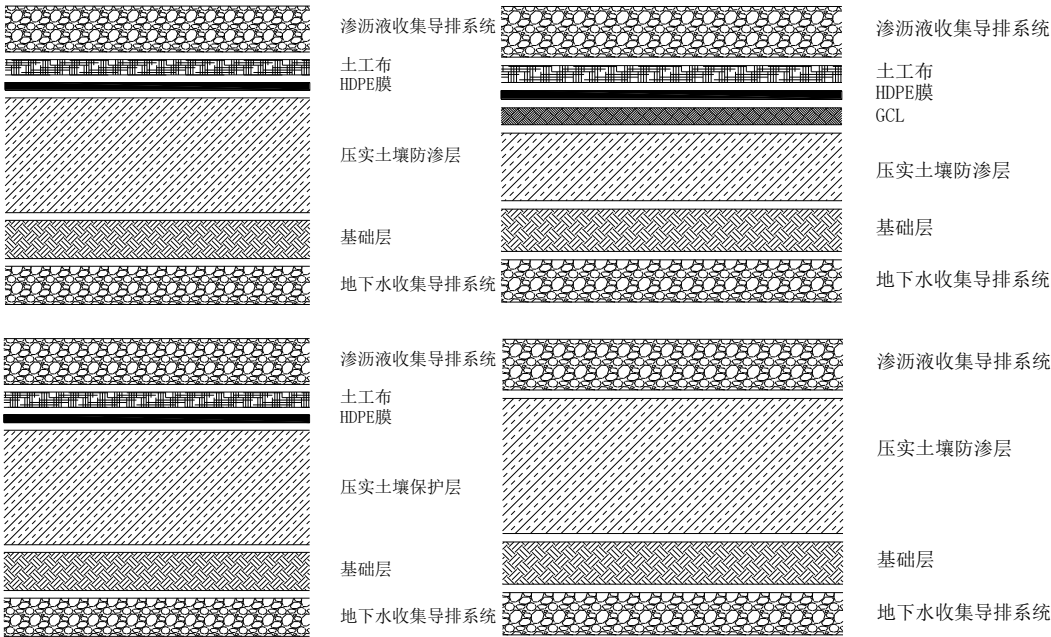
图 4.1-7 单层防渗及单层复合防渗结构的层次
