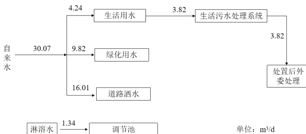
图 3.6-1 现有项目水平衡图
