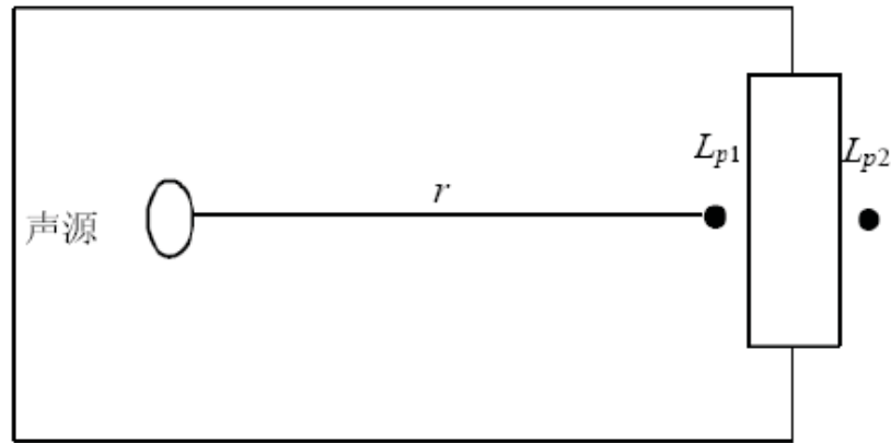
图 6.5-1 室内声源等效为室外声源图例
