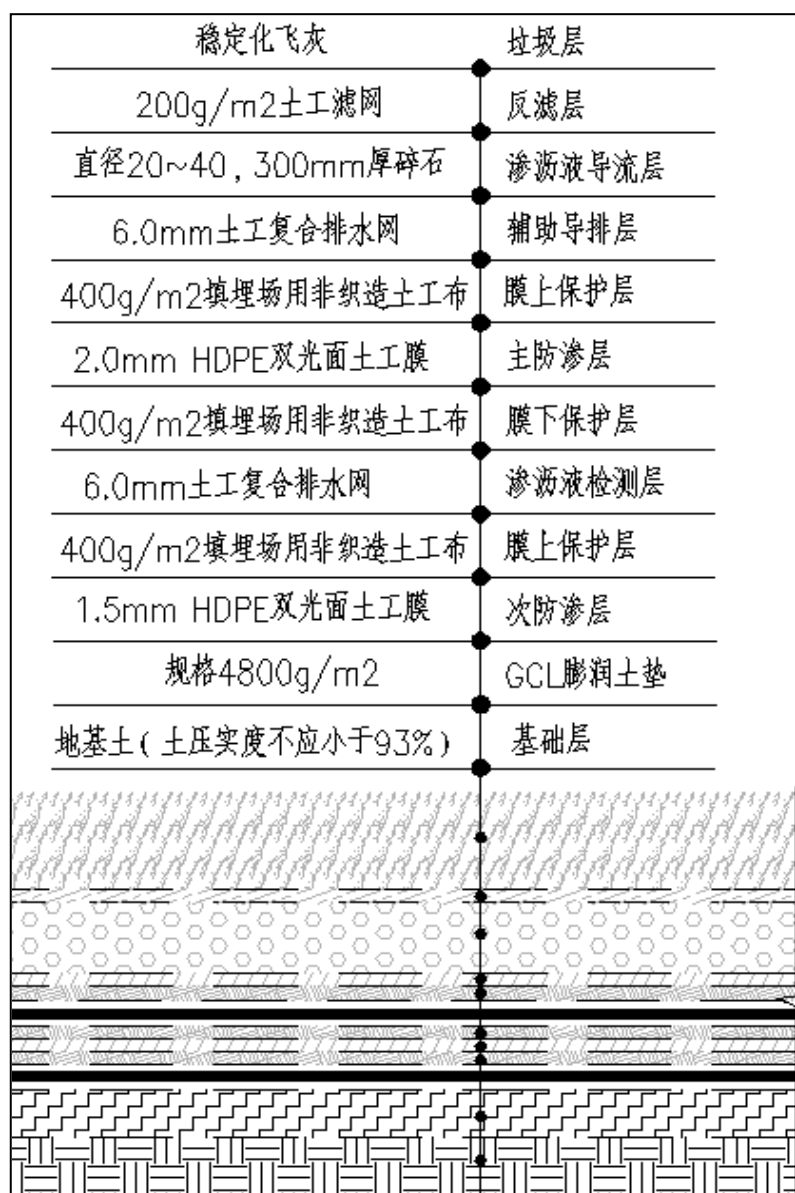
图 7.3-2 库区场底防渗层示意图
