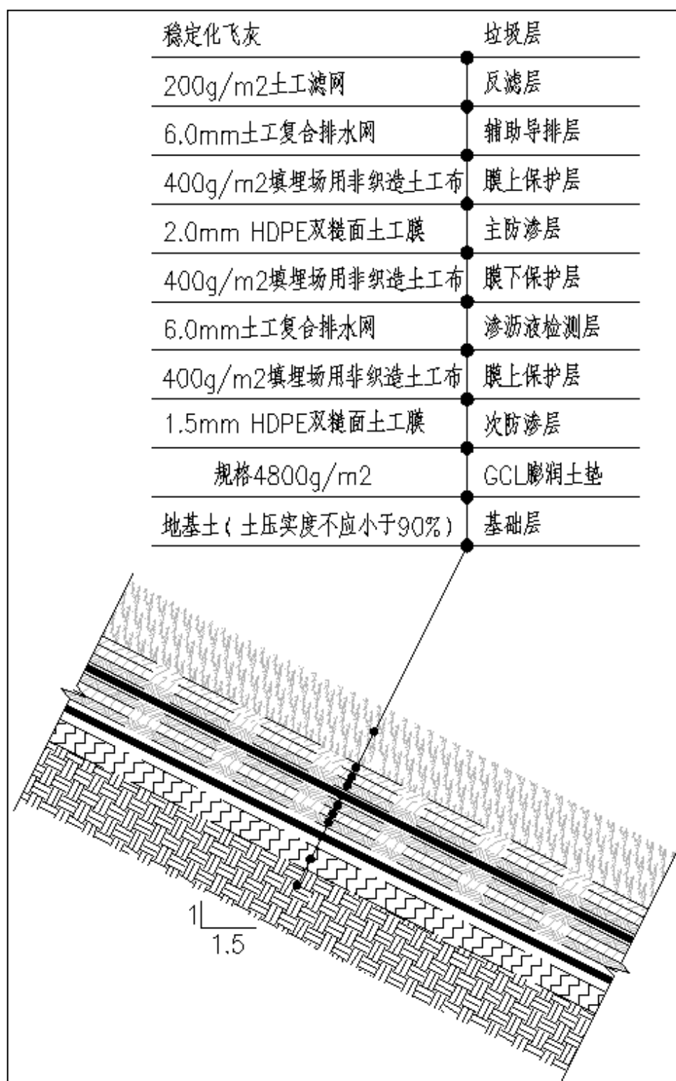
图 7.3-3 库区边坡防渗系统结构图
