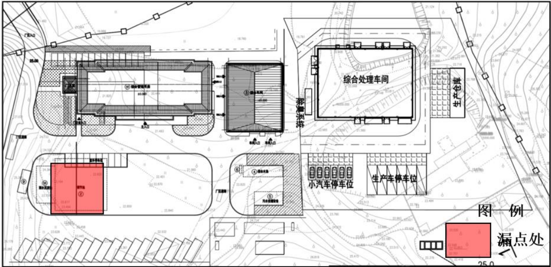
图 6.3-5 地下水泄露点分布图
