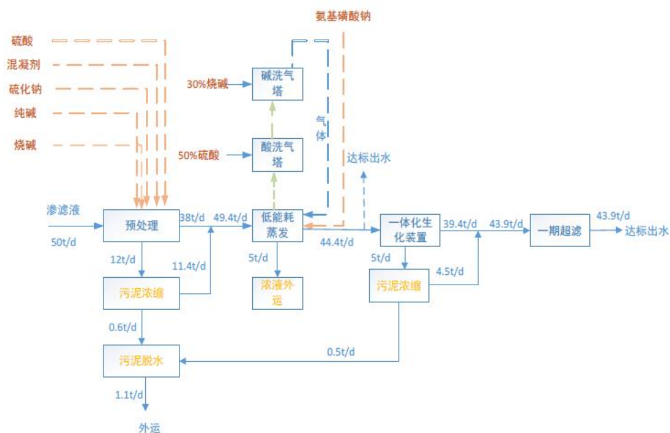
图 3.12-1 淋溶水处理系统改造后工艺流程及水量平衡图
