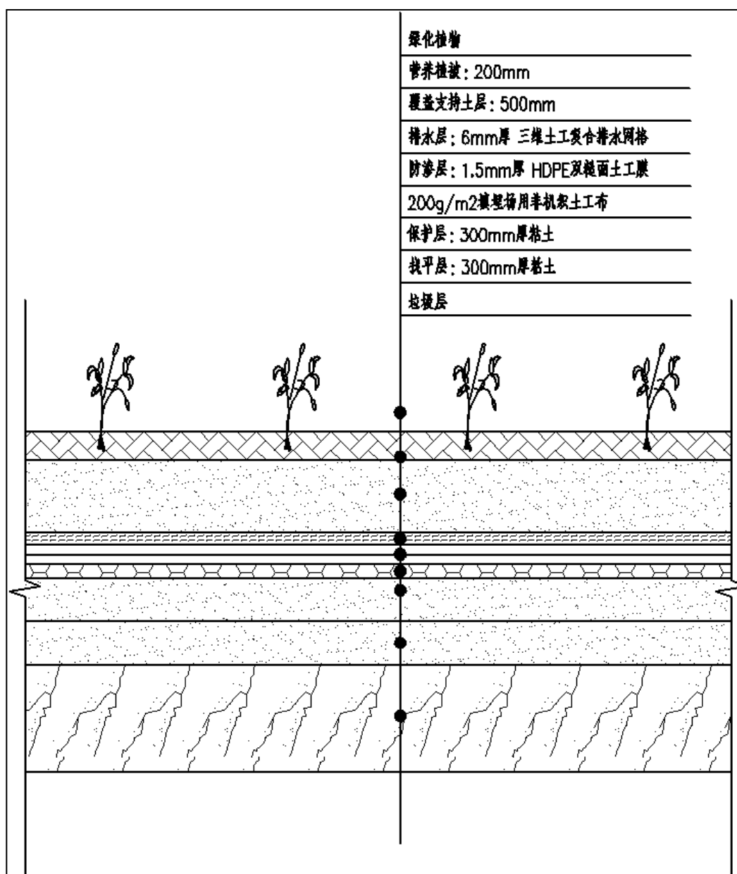
图 7.6-1 标准封顶结构层
